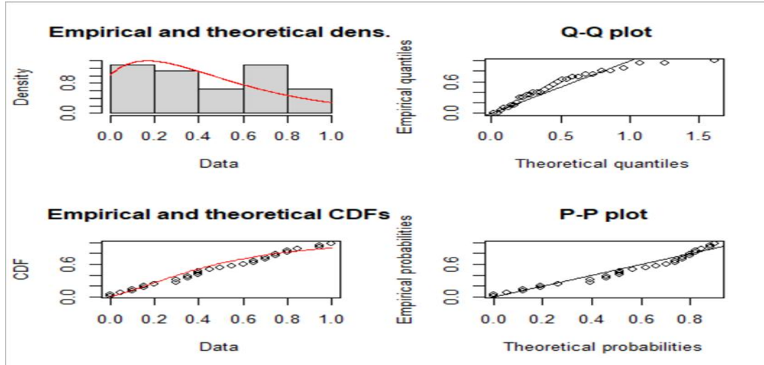
الشكل (2) يمثل دالة الكثافة الاحتمالية ودالة التوزيع التجميعية
