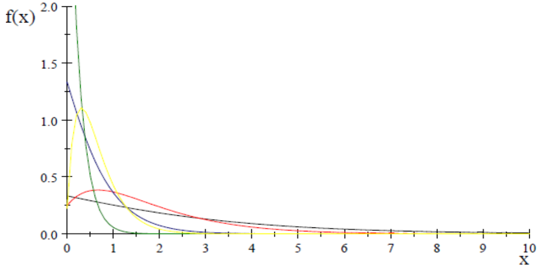
الشكل رقم 1 يمثل دالة الكثافة الاحتمالية لتوزيع كاما ليندلي بمعلمات مختلفة.
