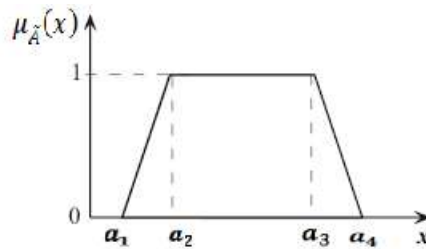
الشكل (3): دالة انتماء شبه المنحرف, [5]
