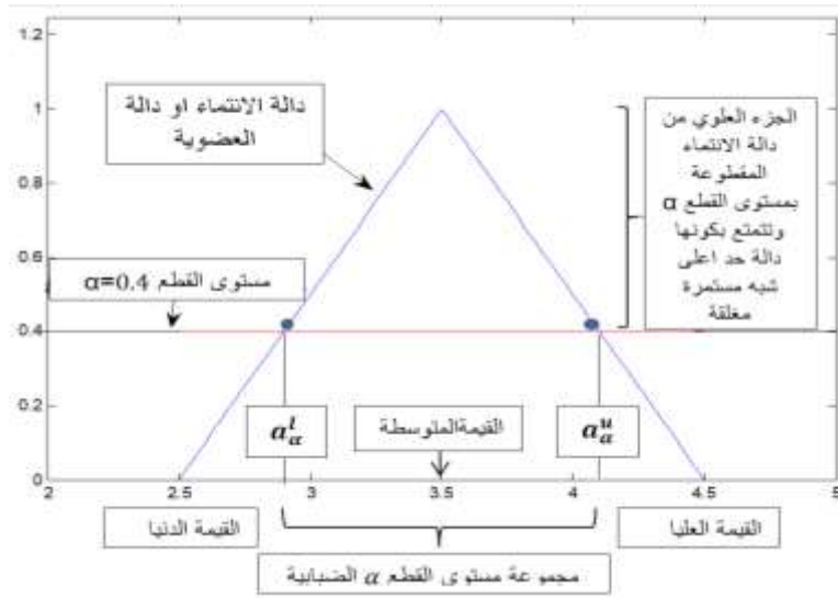
الشكل (7): العدد الضبابي المثلثي بالتفاصيل. المصدر: تم اعداد الشكل من قبل الباحث.
