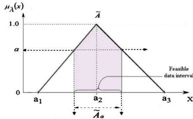
الشكل (4): مستوى القطع \alpha و مجموعة مستوى القطع \tilde{A}_\alpha , [30], [33].
