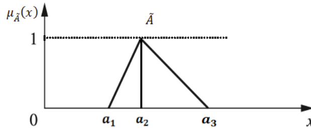
الشكل (2): دالة الانتماء المثلثية, [2], [5]
