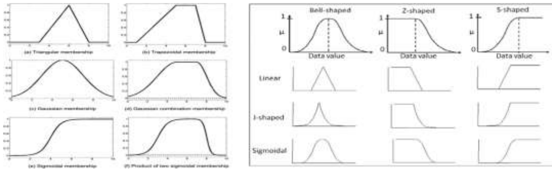
الشكل (1) : انواع منحنيات دوال الانتماء المختلفة, [9],[11]
